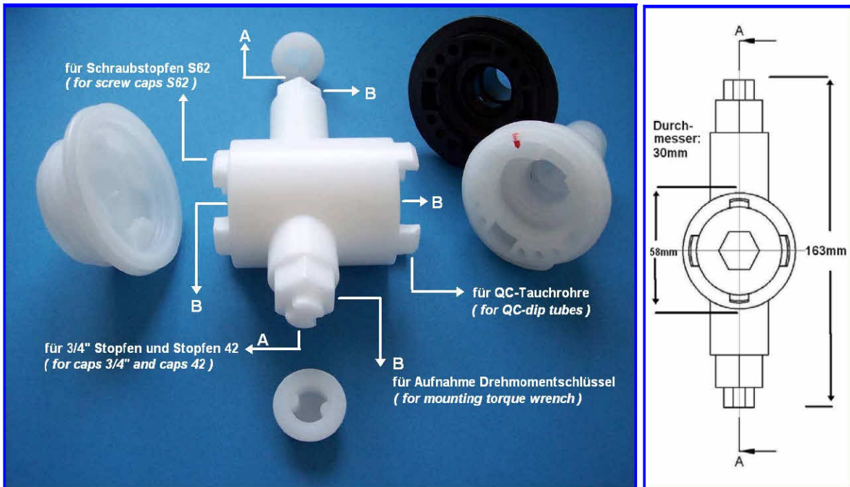
Fass-Schlüssel RDH-79003 zum sicheren Öffnen und Schließen von Tauchrohren mit dem QC-Kopf ( universal wrench RDH-79003 for opening and connecton of dip tubes with the QC-Head )
