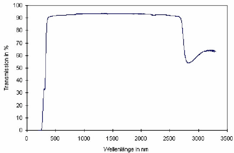
Transmissionsspektrum FOTURAN Glas
