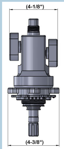
連接接口
